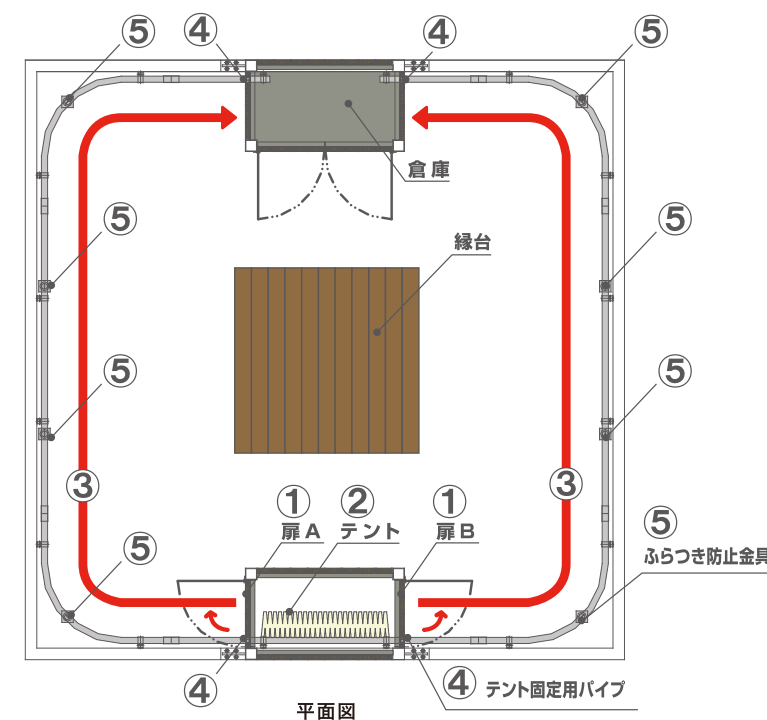
平面図
