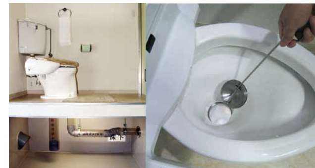
汲み取り式へチェンジする「ハイブリッド便器」と「地下ピット」
