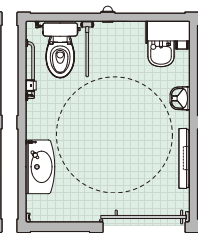
U7型 多1 オストメイト ベビーチェア付 ベビーシート付
