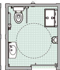
U3型 多1 ベビーシート付 ベビーチェア付
