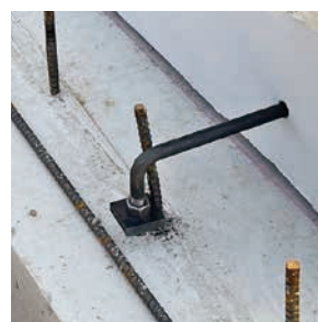
工程 5 基礎へ埋設する部分にL型アンカーを取り付けます。
