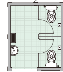
W1型 洋大2 小棚
