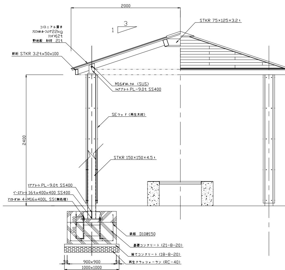
断面図 S=1:20
