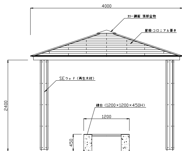
立面図 S=1:30
