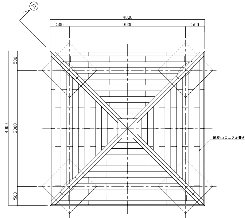
平面図 S=1:30
