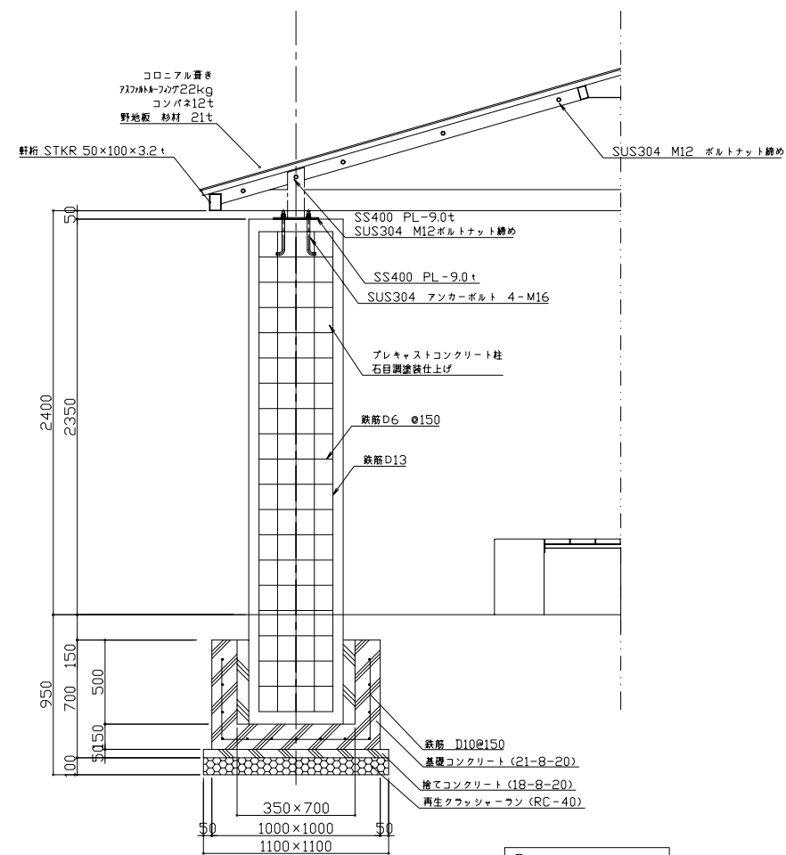
① 断面図 S=1:20
