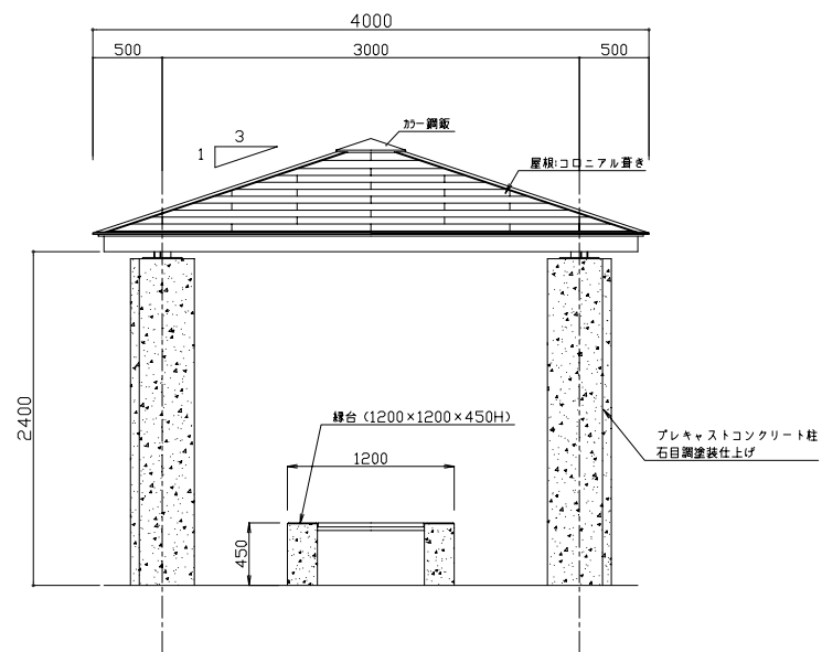
立面図 S=1:30
