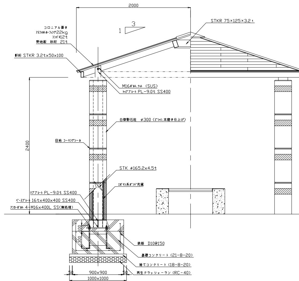
断面図 S=1:20
