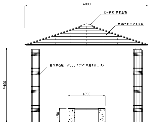
立面図 S=1:30
