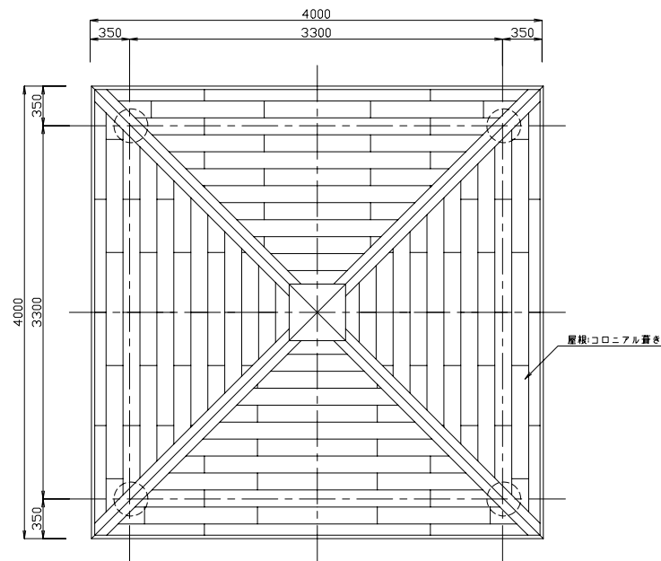
平面図 S=1:30
